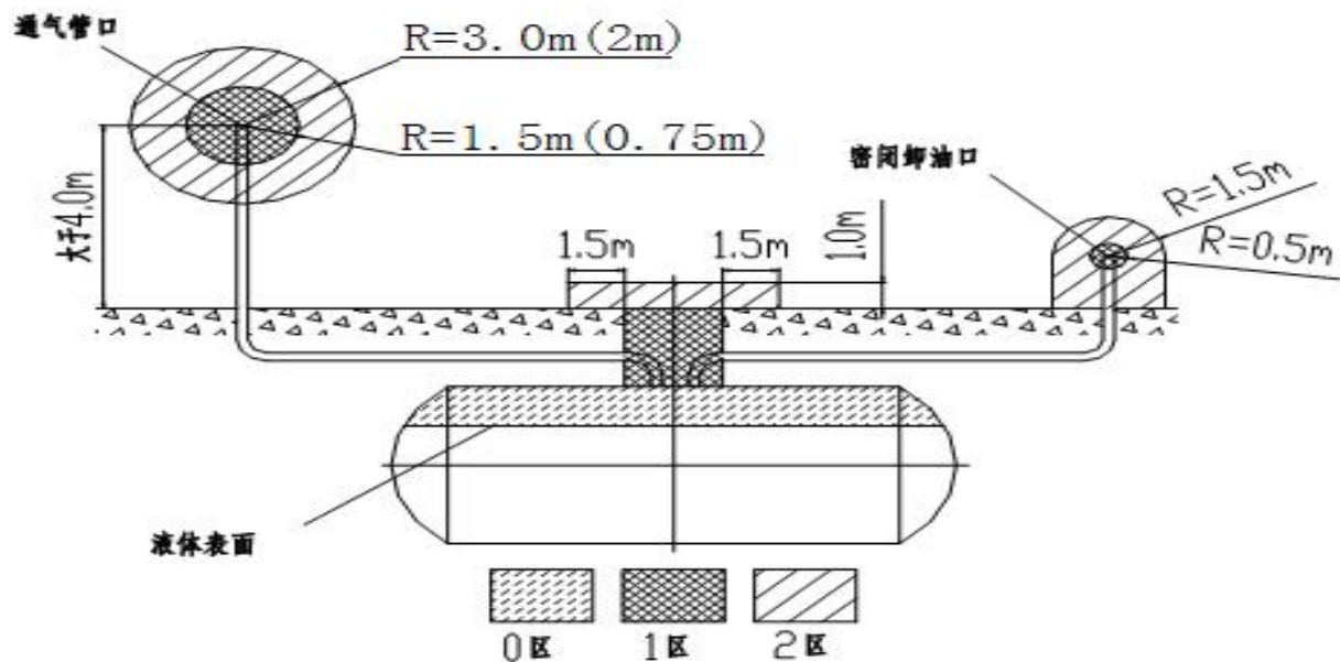
图 3.4-1 埋地卧式油罐的爆炸危险区域划分图
