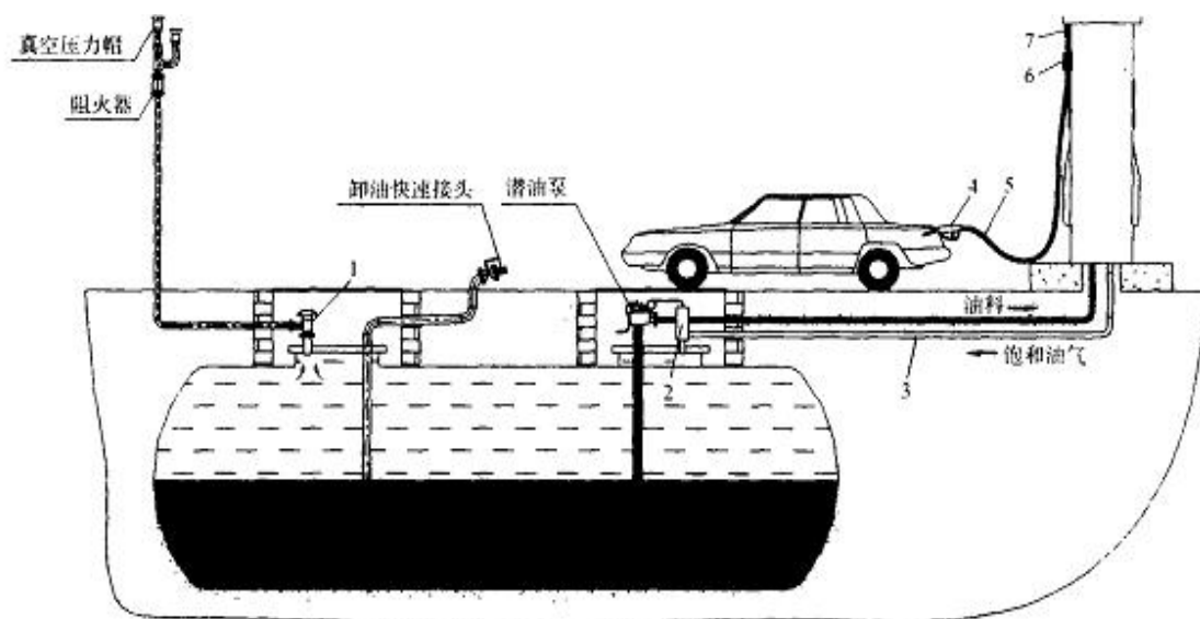
图 2.5-2 加油油气回收系统示意图
